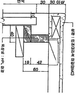
"B" : 하부장 상판 돌코 & 손잡이 상세
