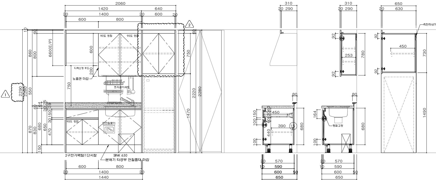
ELEVATION
