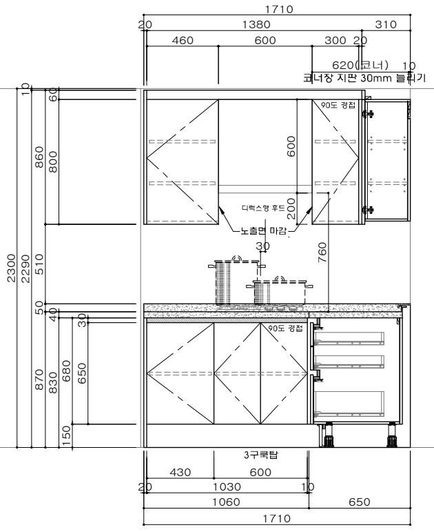
B ELEVATION
