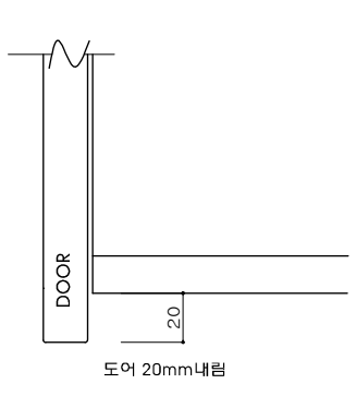
상부장 손잡이 상세
