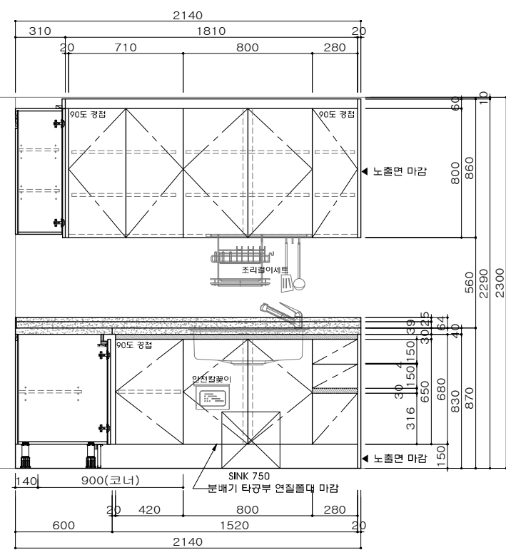
A ELEVATION
