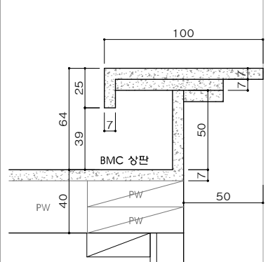
하부장 뒷선반 상세
