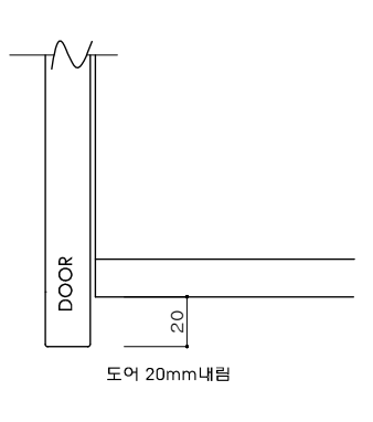
상부장 손잡이 상세
