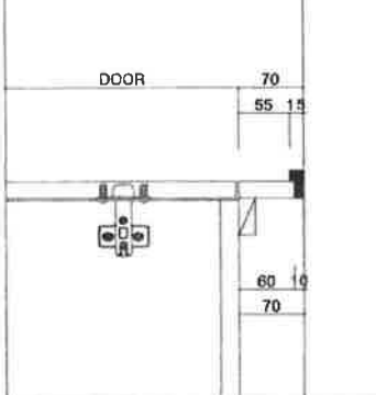
■ 상부 물림 상세도
