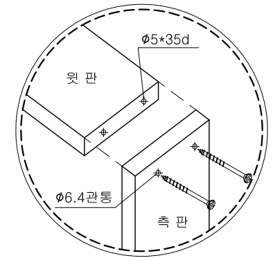
< 문틀 조립도 >
