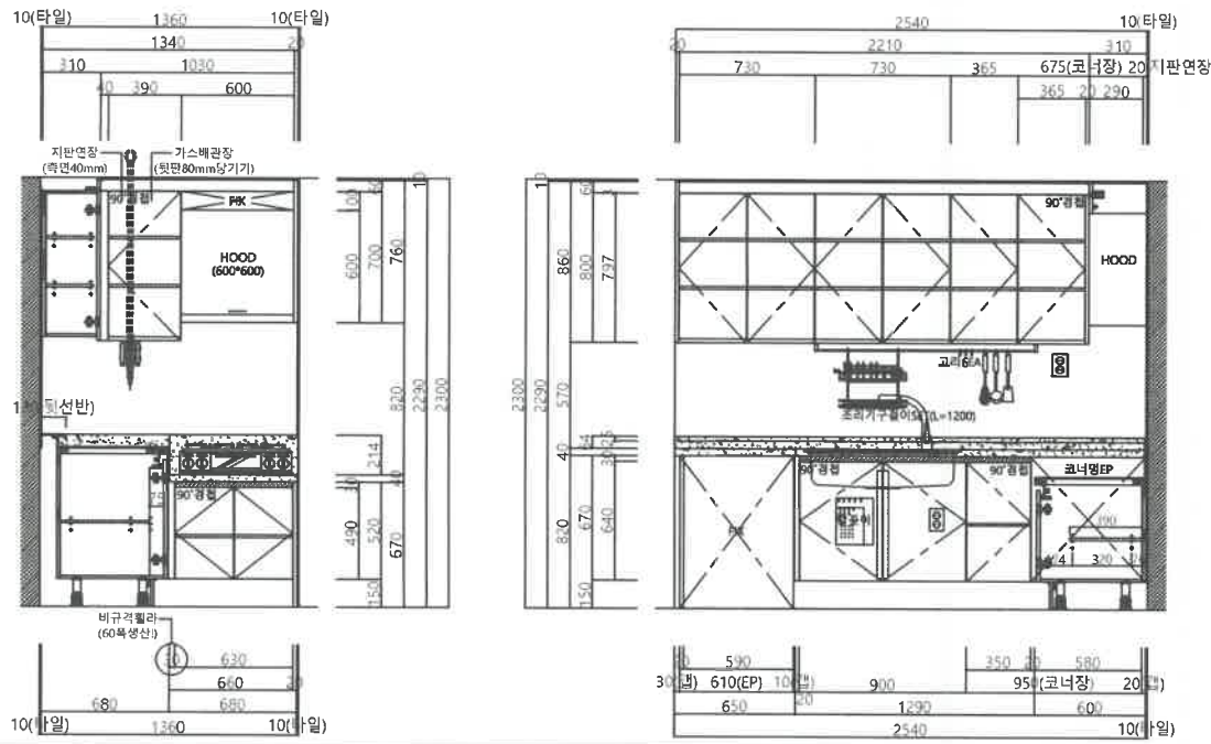
ELEVATION - A
