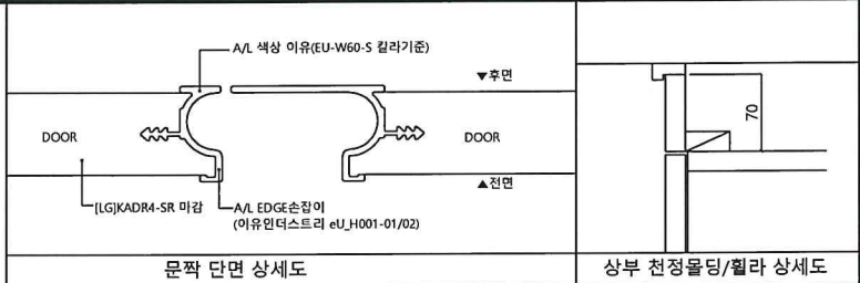
문짝 단면 상세도
