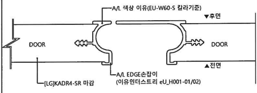
문짝 단면 상세도
