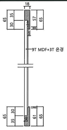
문경 상하단면 상세도
