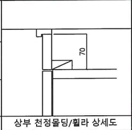
상부 천정돌림/휠라 상세도
