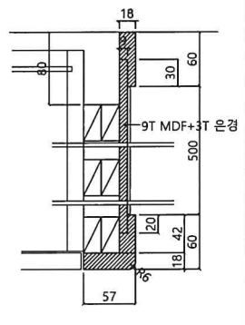
문경 좌우단면 상세도
