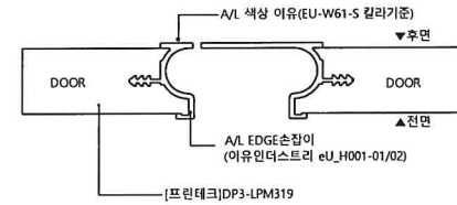
문짝 단면 상세도
