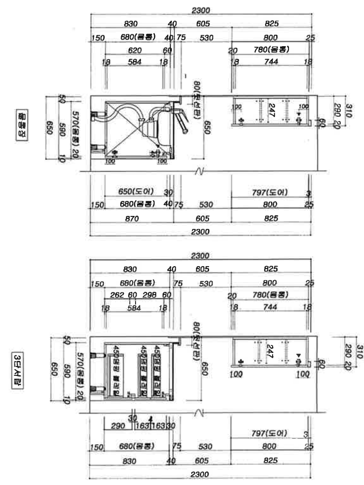
단면도-A
