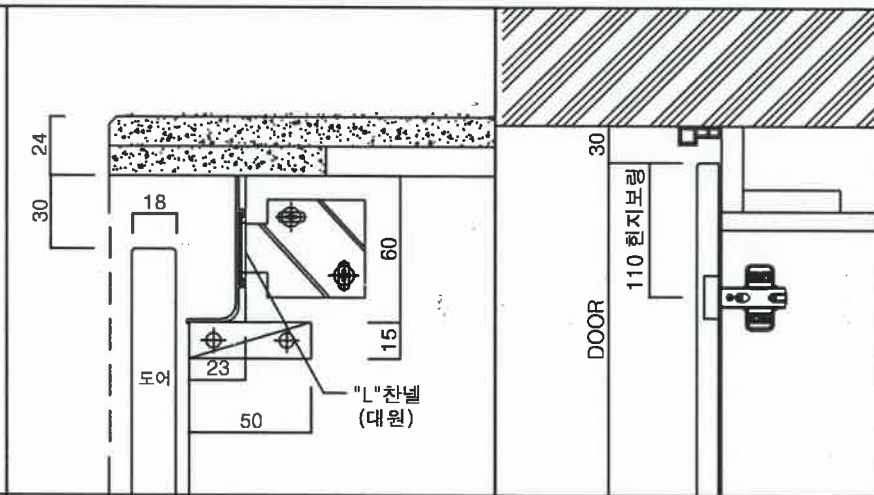
하부장 DOOR DETAIL
