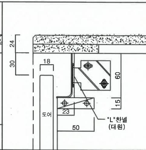
하부장 DOOR DETAIL
