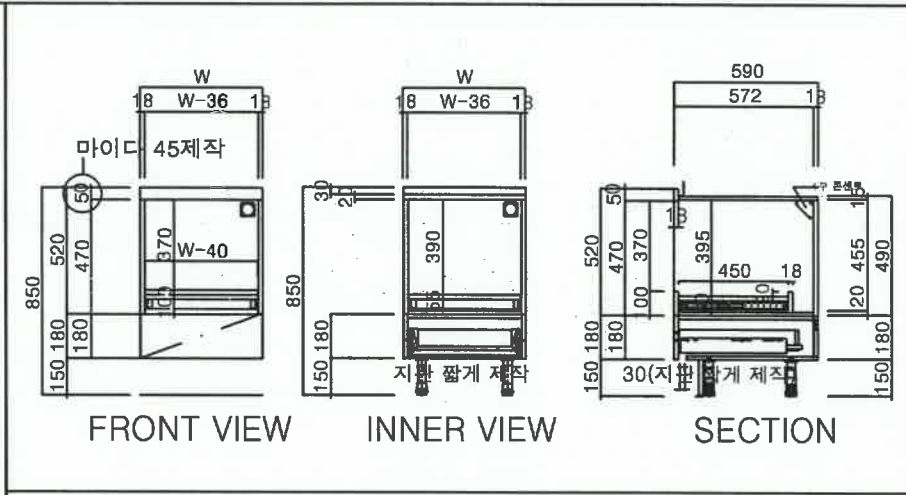
밥통장 DETAIL
