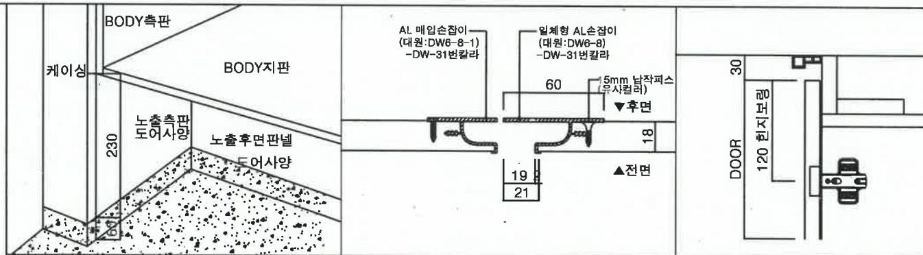
하부 오픈부 DETAIL
