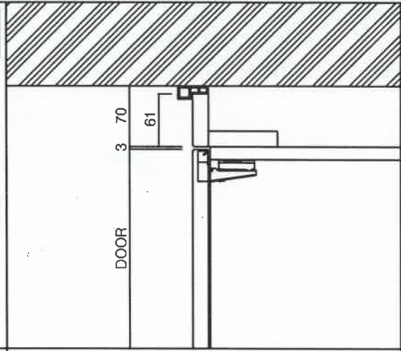
냉장고 상부 MOULDING DETAIL
