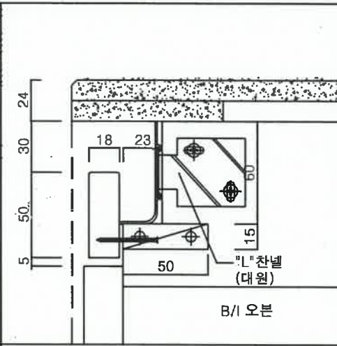
하부장 DOOR DETAIL(오븐)
