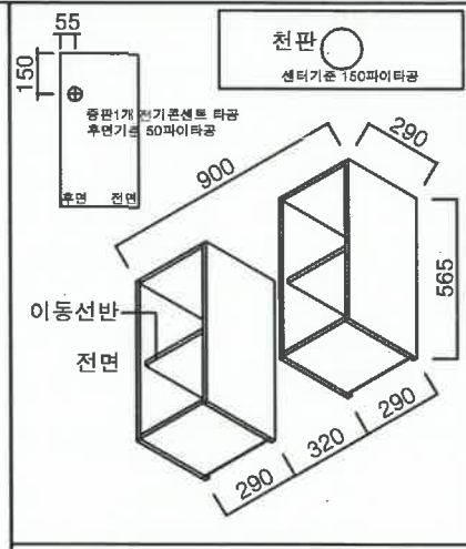
후드장 상세도
