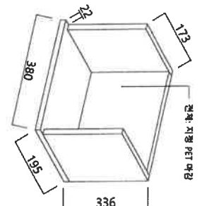
오른쪽 치면 전면(DMM) 키우기 오른쪽 치면 전면(입식형)
