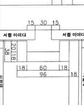
서랍장 손잡이 상세도
