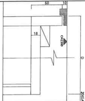
상부 코니스 상세도
