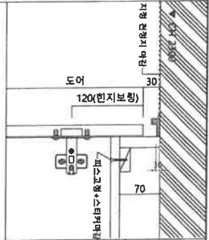
상부 코너스 상세도
