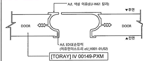
문짝 단면 상세도
