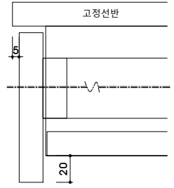
내부서랍 DETAIL
