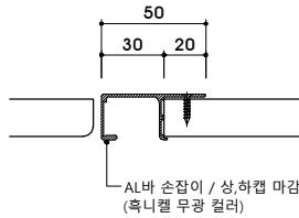
도어손잡이 DETAIL
