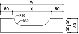
도어손잡이 DETAIL
