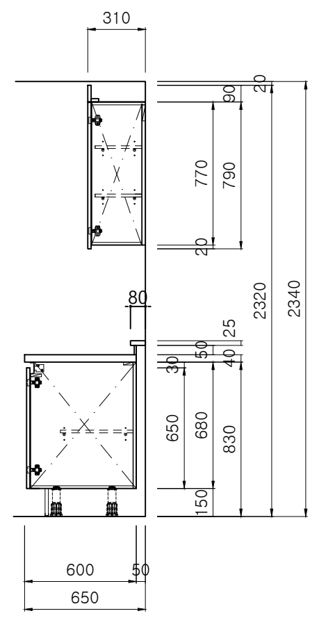
하부장 목찬널 DETAIL 'B'
