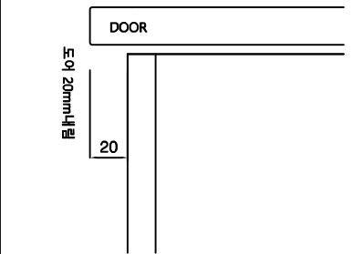
상부장 손잡이 DETAIL
