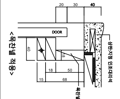
하부장 손잡이 DETAIL
