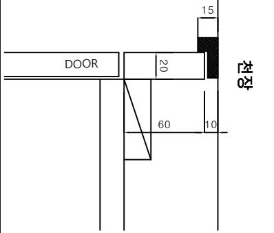
상부 휠라 DETAIL
