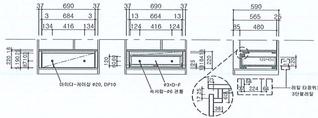
내부서랍 상세도 / 조절나사 설치
