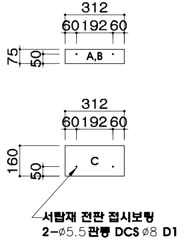
서랍재 전판 보링도
