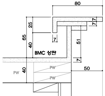
하부장 뒷선반 상세
