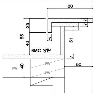
하부장 뒷선반 상세
