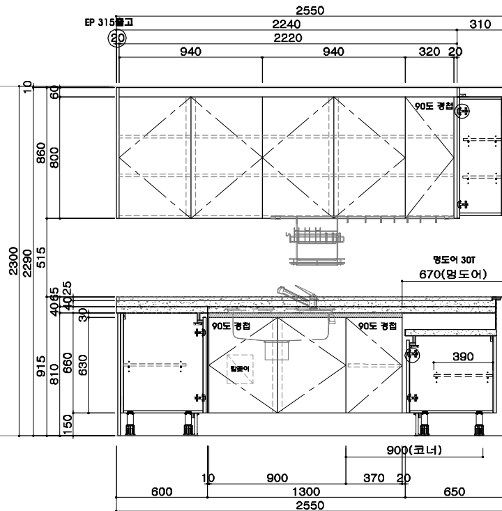
A ELEVATION
