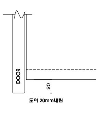
상부장 손잡이 상세
