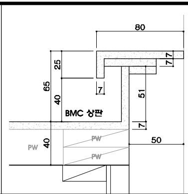
하부장 뒷선반 상세
