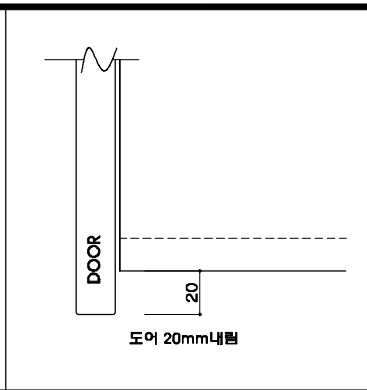
상부장 손잡이 상세
