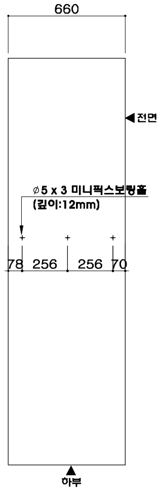
우 E/P판
