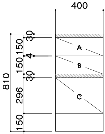
입면도
