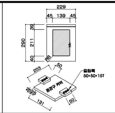
점검수 상세
