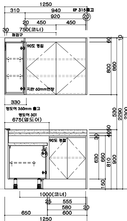
B ELEVATION
