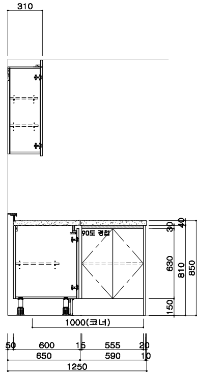
B ELEVATION
