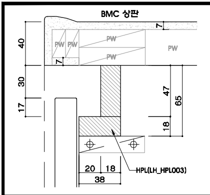
하부장 손잡이 상세
