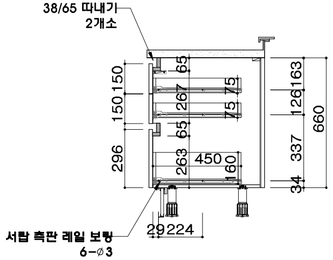
측면도
