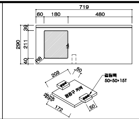
점검수 상세
