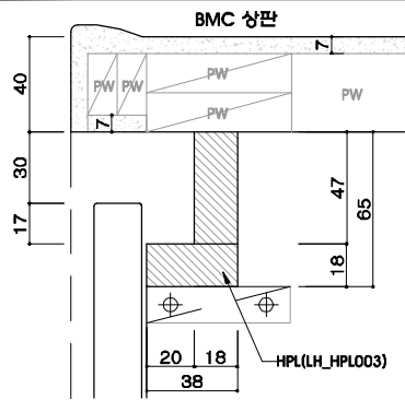
하부장 손잡이 상세
