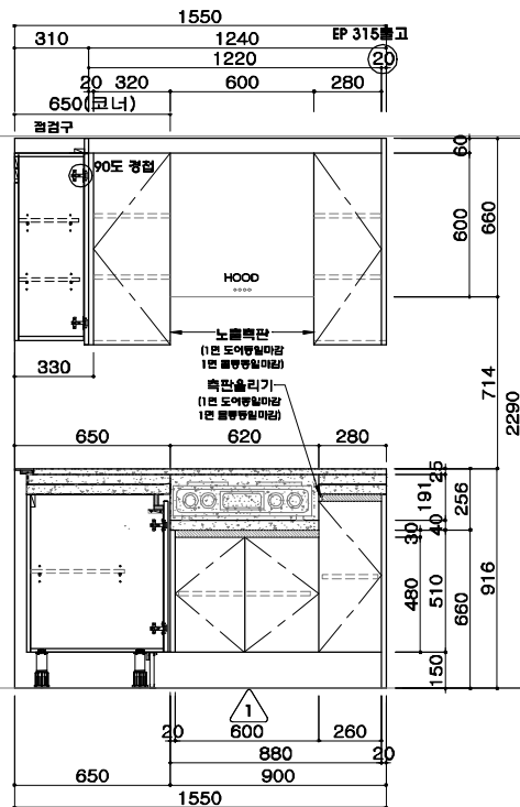
B ELEVATION
