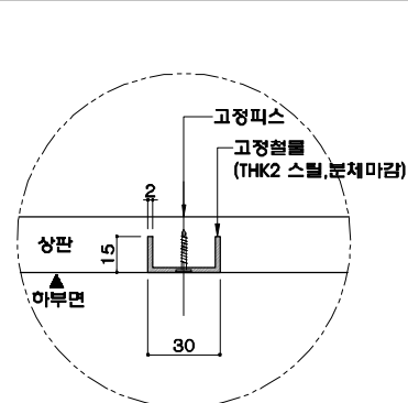
"A" 상세(상판철물보강)
