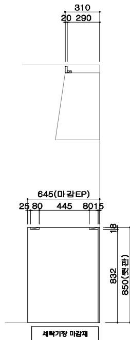
세탁기장 마감재
