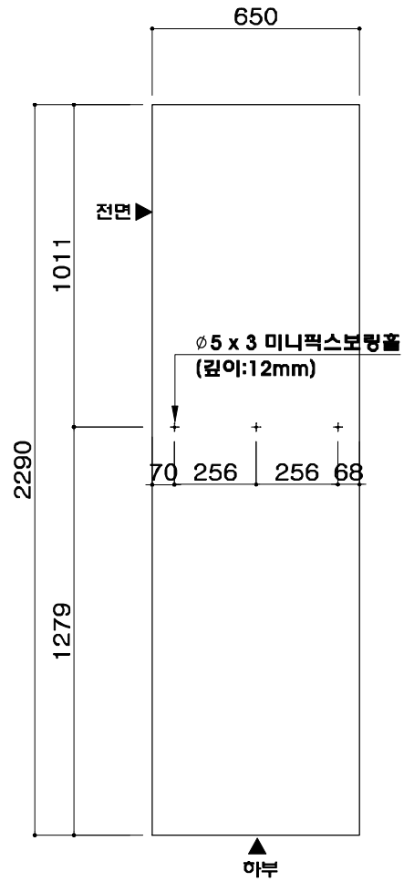
좌 E/P판
