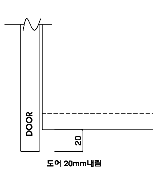
상부장 손잡이 상세
