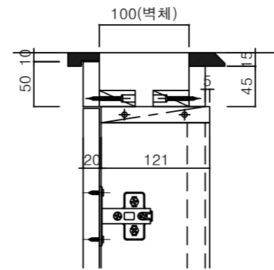
문틀 상세도
