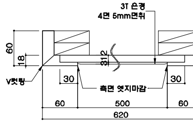
측면 경 DETAIL
