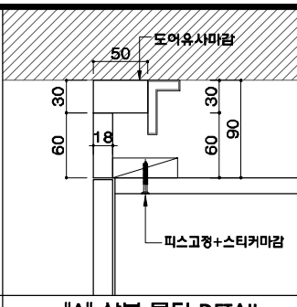
"A" 상부 물뎡 DETAIL
