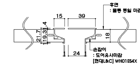
손잡이 DETAIL
