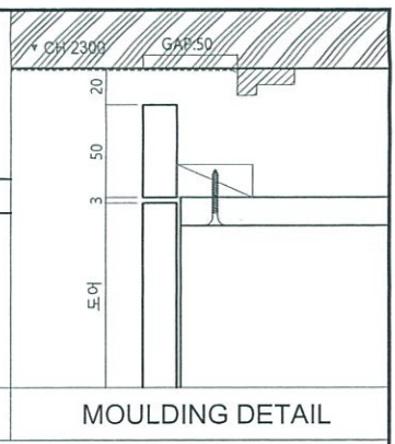
DOOR DETAIL
