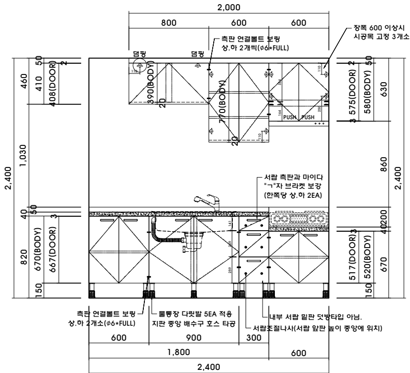
2 ELEVATION-A
