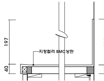
DETAIL2 : BMC 상판(가스대)
