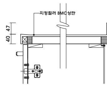
DETAIL1 : BMC 상판(LH사양으로 제작 요망)
