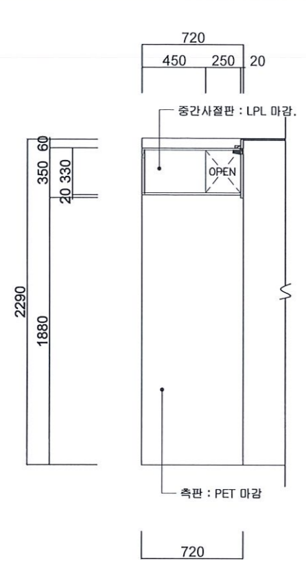
E 84㎡A형 주방가구 냉장고장 측면도
