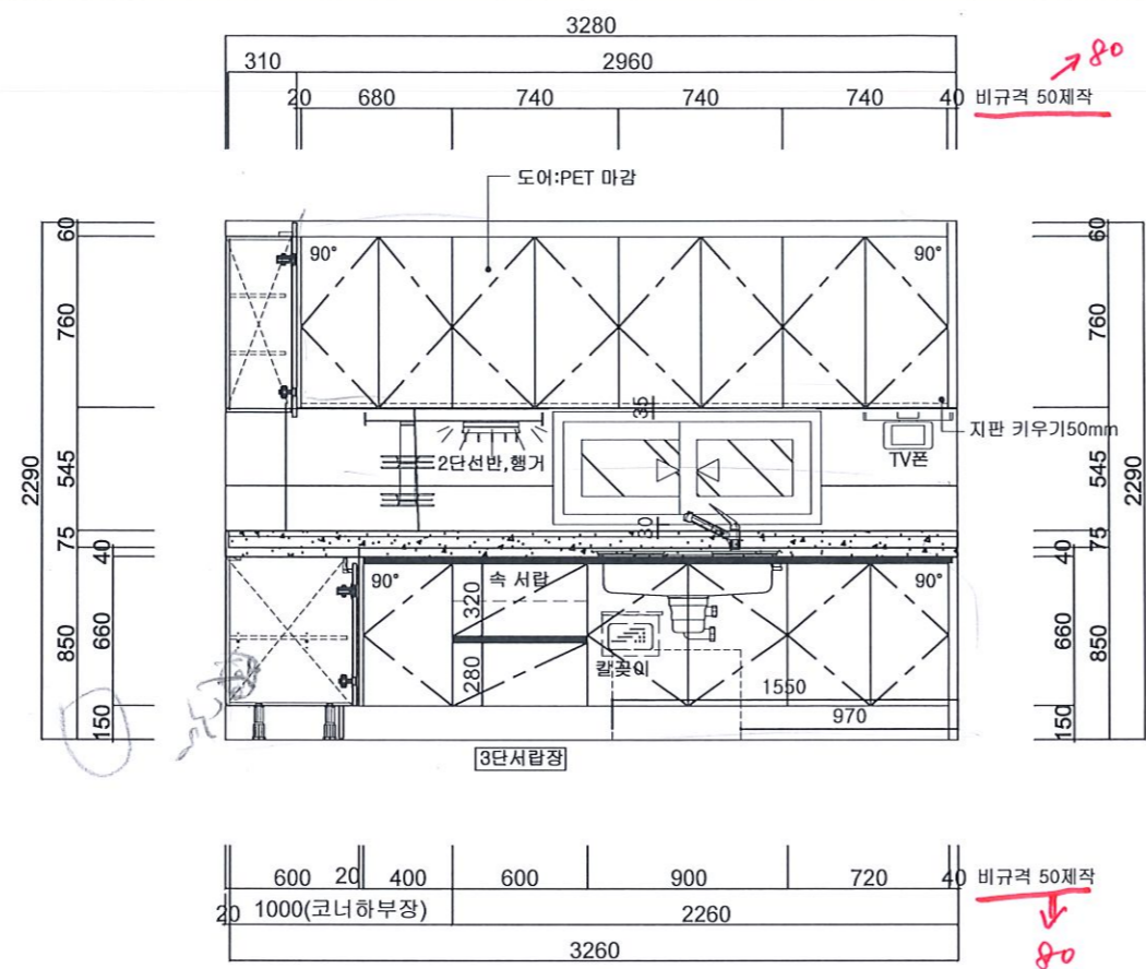
B 84㎡A형 단위세대 주방가구 입면도
