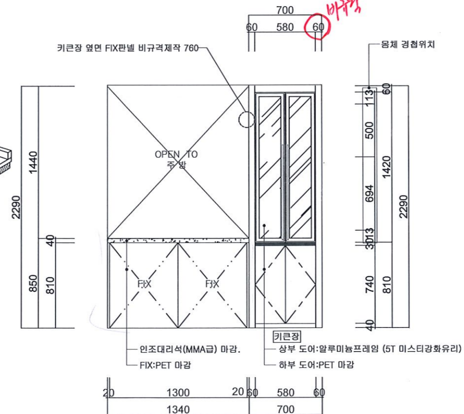
E 74㎡A형 단위세대 주방가구 입면도
