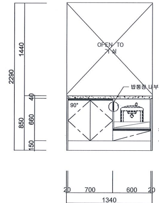
C 74㎡A형 단위세대 주방가구 입면도
