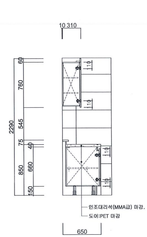
D 84㎡A형 단위세대 주방가구 입면도
