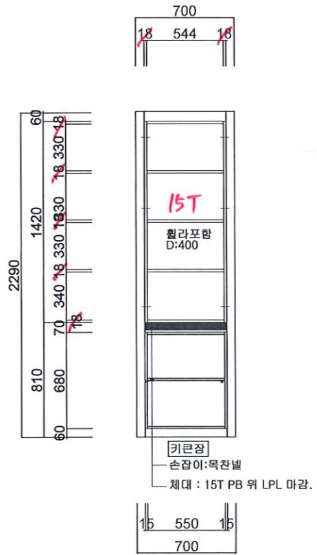
E 내부도
