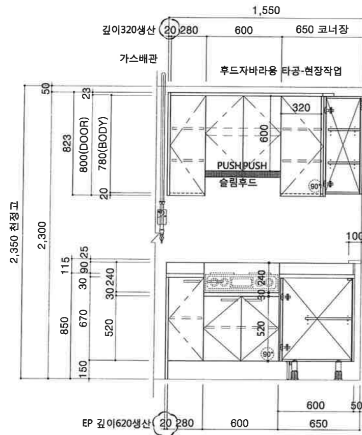
ELEVATION-A
