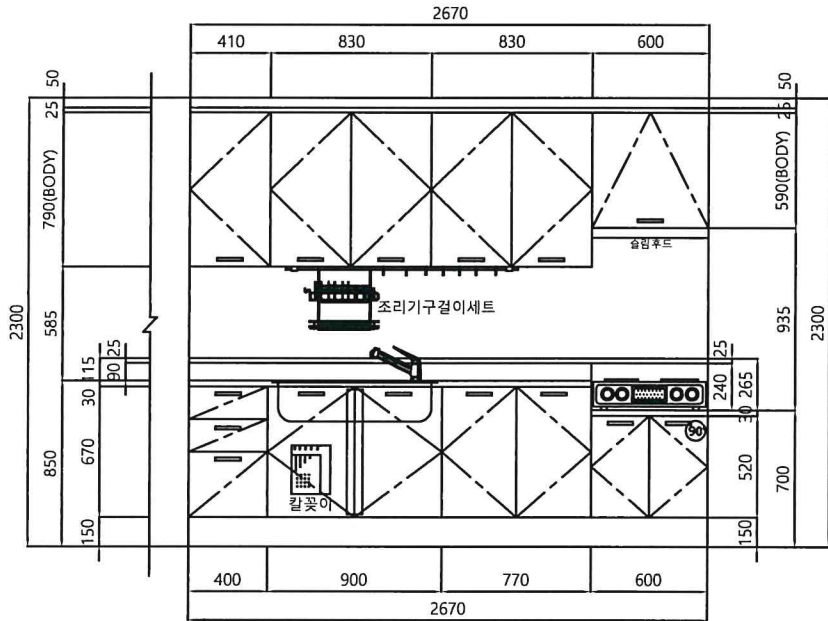
입면도 A
