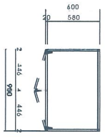
정면도
