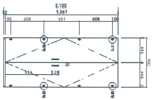
정면도
