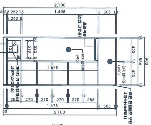
내부도
