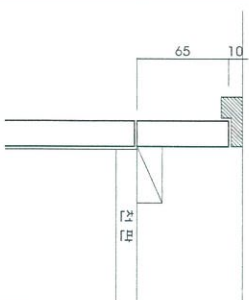
상부웨사 DETAIL
