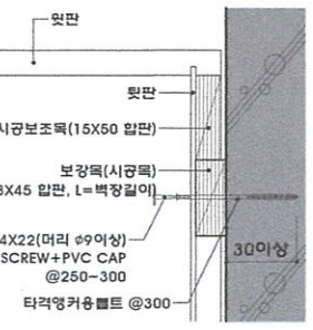
4 부분 상세
