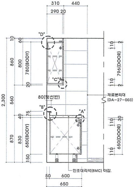
2 마감사항 및 부분 상세
