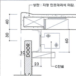
"B" : 하부장 뒷선반 상세
