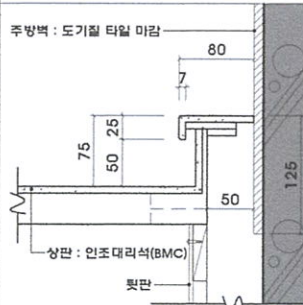
2 마감사항 및 부분 상세
