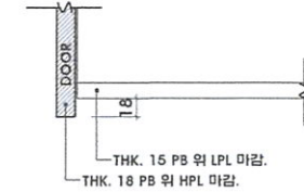
"C" : 상부장 손잡이 상세
