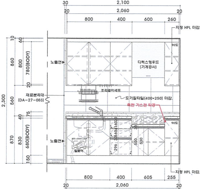
3 주방가구 입면도 A, B
