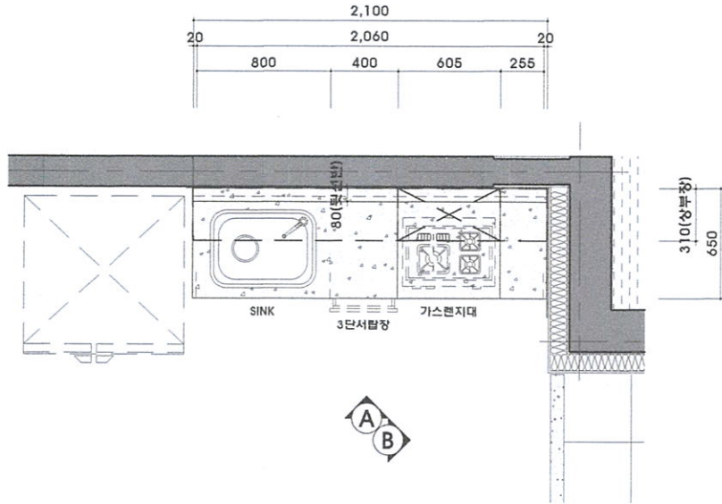
1 26A, 29A형 단위세대 주방가구 평면도
