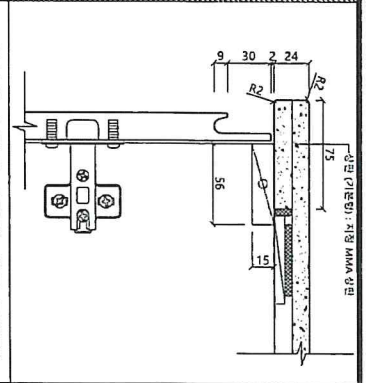
하부장 손잡이 디테일 (상판 기보형)
