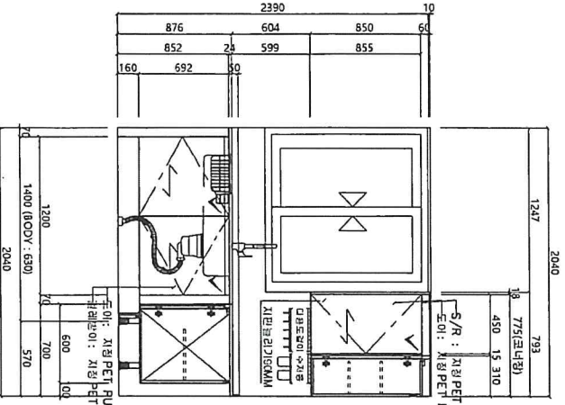
A ELEVATION
