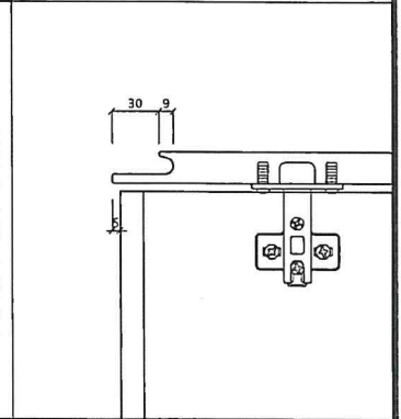
상부장 손잡이 상세도
