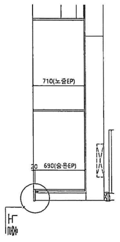
상부장 몸뚱이 상세도
