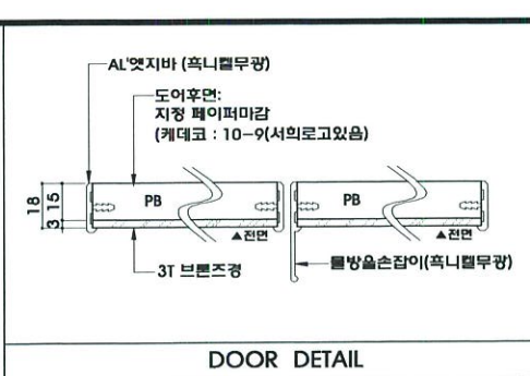
DOOR DETAIL
