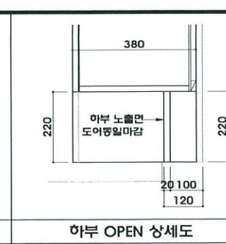
하부 OPEN 상세도
