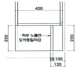
하부 OPEN 상세도
