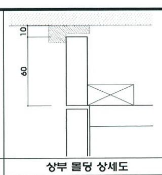
상부 풀딩 상세도
