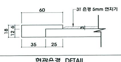
현관은경 DETAIL
