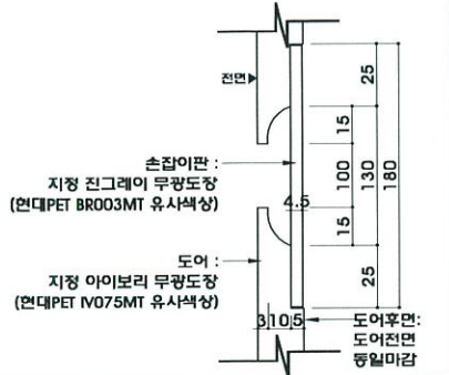
DOOR DETAIL
