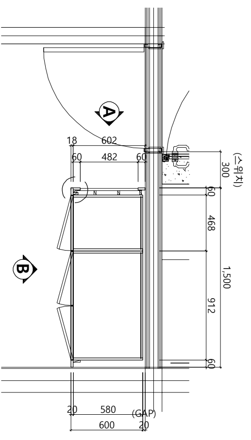
평면도
