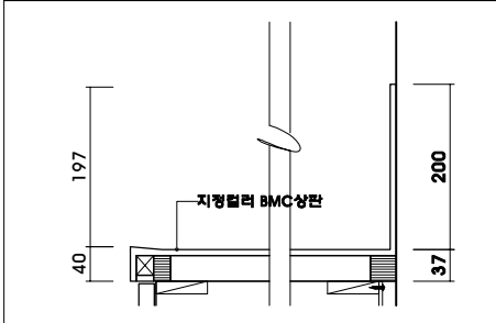
DETAIL2 : BMC 상판(가스대)
