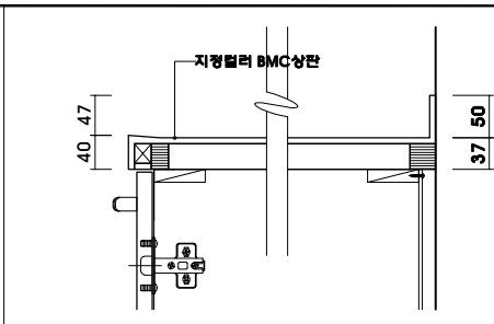
DETAIL1 : BMC 상판(LH사양으로 제작 요망)
