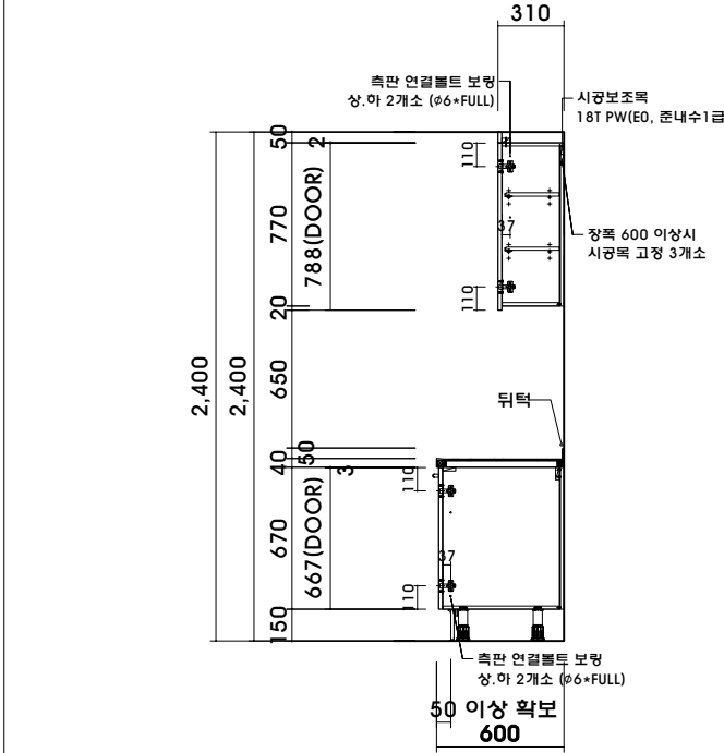
DETAIL2 : BMC 상판(가스대)
