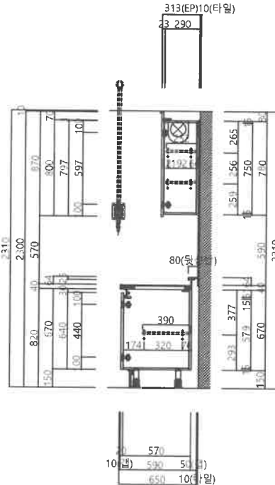
SIDE SECTION - 상,하부장
