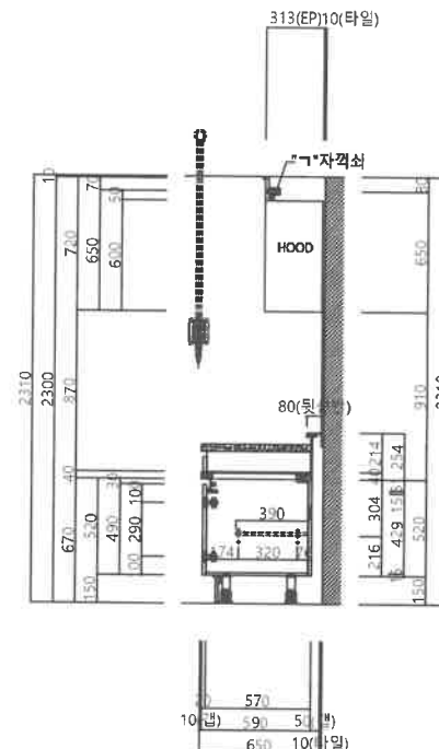
SIDE SECTION - 후드장,가스대
