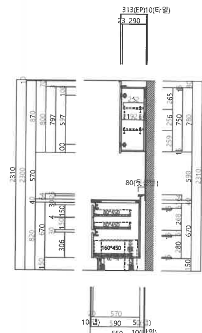
SIDE SECTION - 3단서랍장
