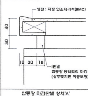
밥통장 마감잔널 상세'A'
