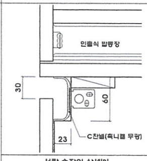
서랍 손잡이 상세'B'
