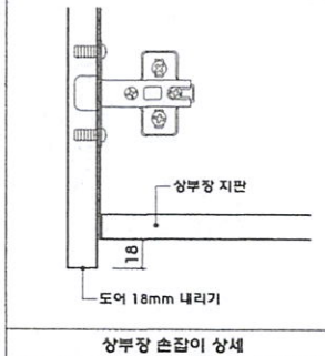
상부장 손잡이 상세
