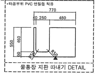
SB장 분배기 가림막 DETAIL
