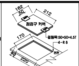
상부 점검구 DETAIL
