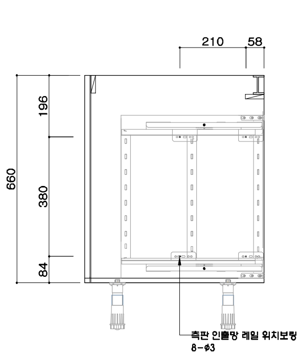
-측판 보링도-
