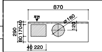
후드장 천판 타공도
