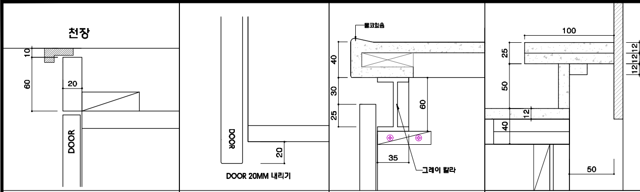
상부활라 DETAIL
