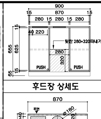
후드장 상세도
