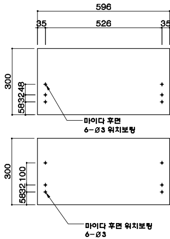
마이디 보강도
