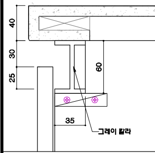
하부장 손잡이 DETAIL
