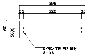
마이다 보링도
