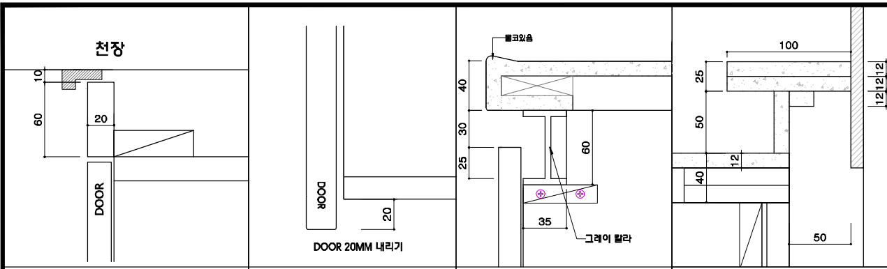
상부활라 DETAIL
