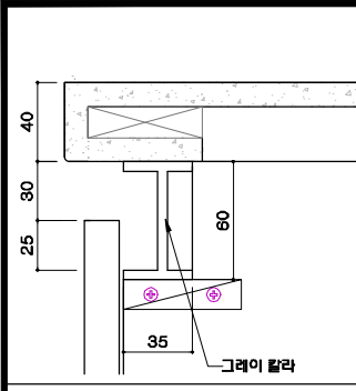
하부장 손잡이 DETAIL
