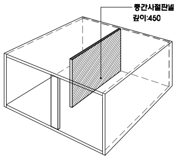
냉장고장 상부장 DETAIL
