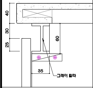
하부장 손잡이 DETAIL
