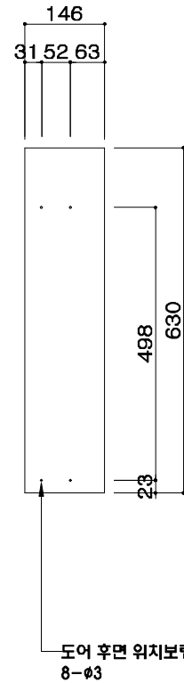
-도어 보링도-
