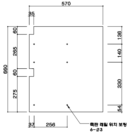
측판보강도
