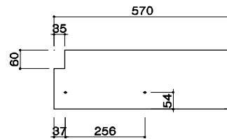
측판보링도
