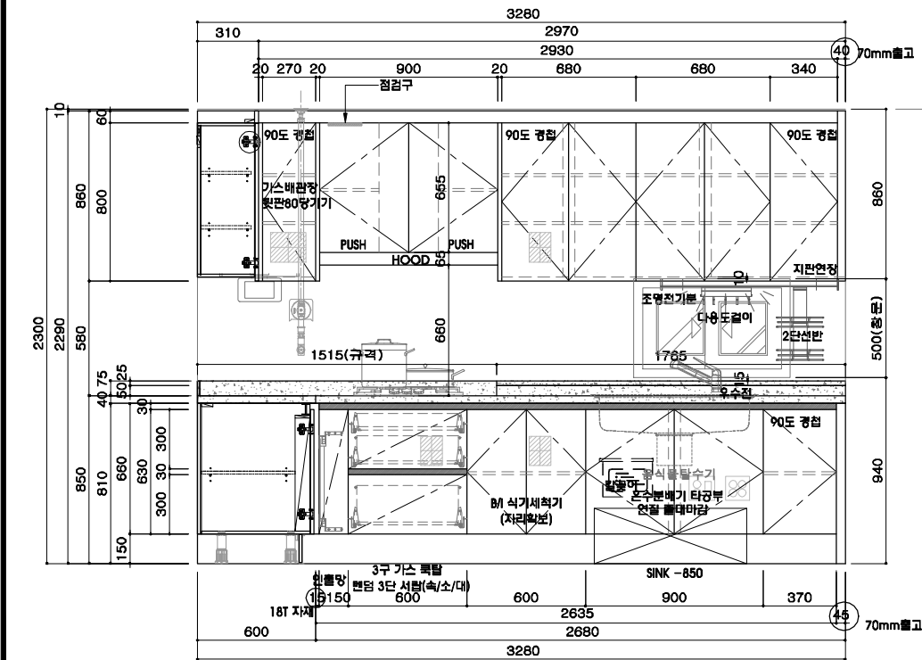
후드장 천판 타공도
