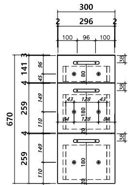
DETAIL2 : BMC 상판(가스대)
