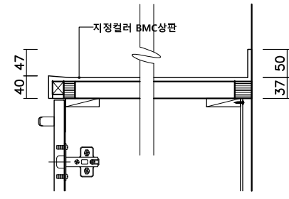
DETAIL1 : BMC 상판
