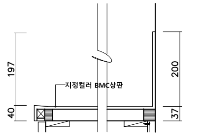
DETAIL2 : BMC 상판(가스대)
