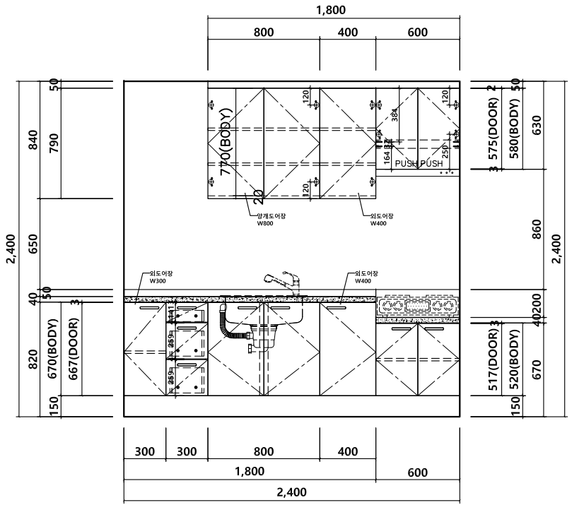
2 ELEVATION-A
