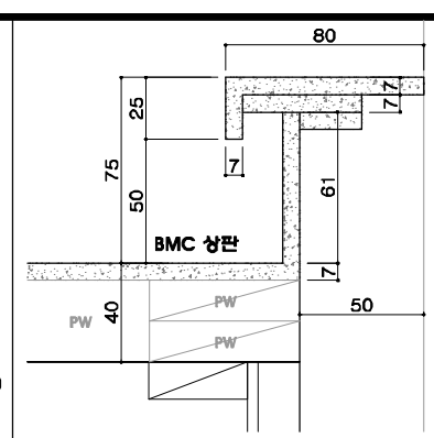
하부장 뒷선반 상세
