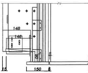
(옵션)오븐장+후라이팬서랍장 상세도
