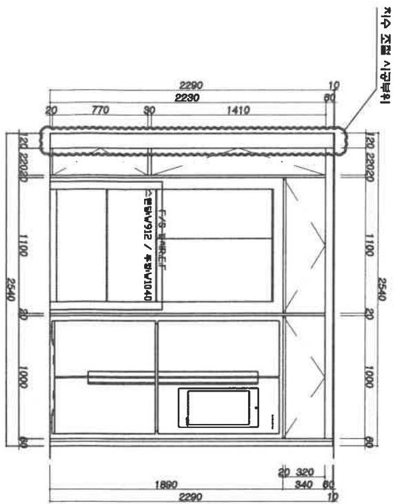
2 입면도-B
