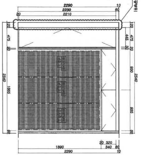
3 입면도-B(냉장고 옵션)(비스포크)
