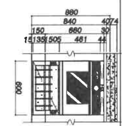
(옵션)오븐장+후라이팬서랍장 상세도
