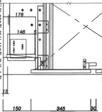
1단서랍장+후라이팬서랍장 상세도
