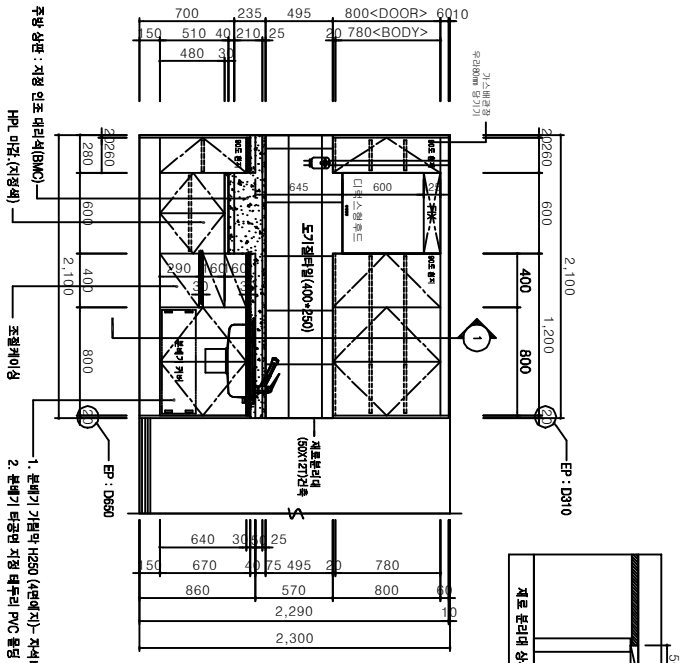
1 26㎡ A형 단위세대 주방기구 평면도
