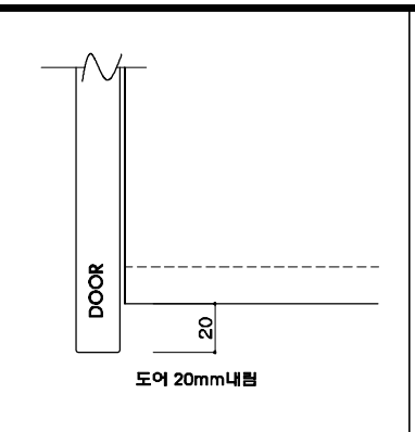
상부장 손잡이 상세
