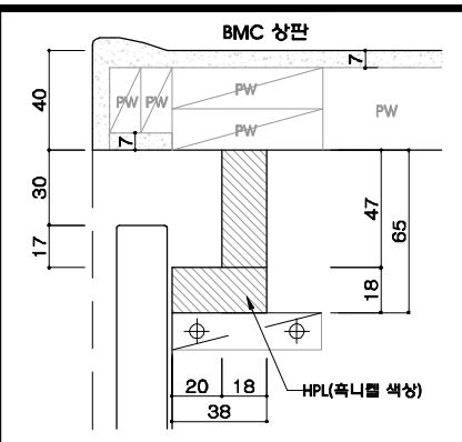
하부장 손잡이 상세
