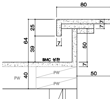
하부장 뒷선반 상세도
