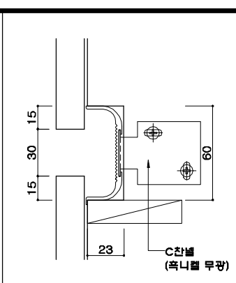
"A" 상세도
