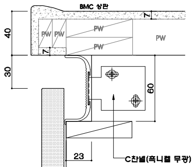
하부장 손잡이 상세도
