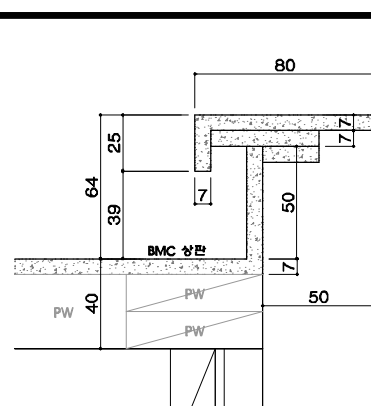
하부장 뒷선반 상세도
