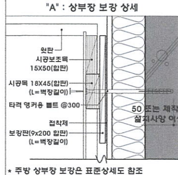
2 주요자재사항 & 부편상세도
