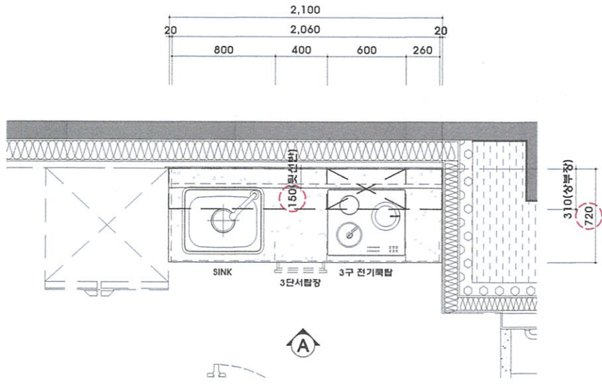
1 26m² A형 단위세대 주방가구 평면도
