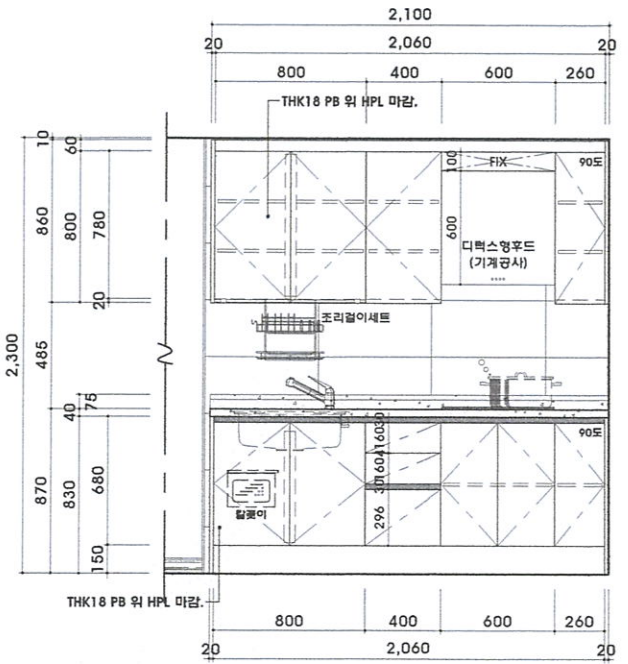
3 주방가구 입면도 A, 측단면도 A
