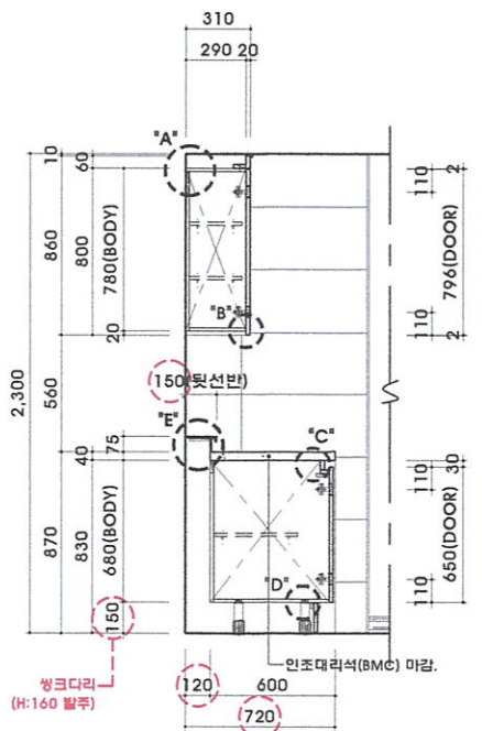
3 주방가구 입면도 A, 측단면도 A
