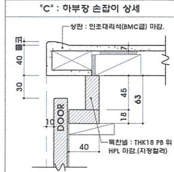
4 상세도
