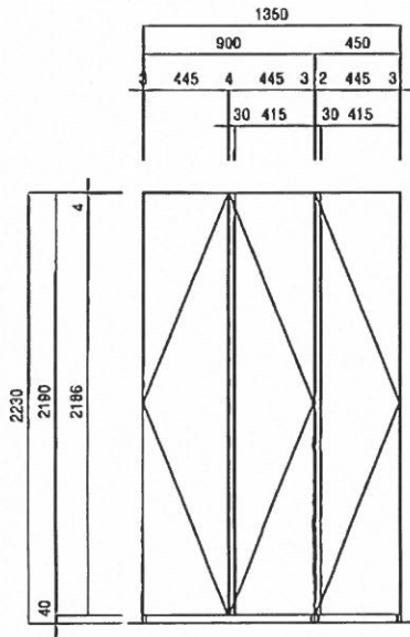
정면도
