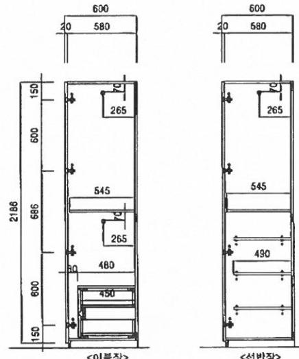
측단면도
