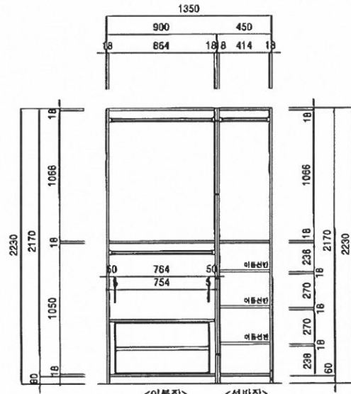
내부도
