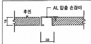
손잡이 DETAIL
