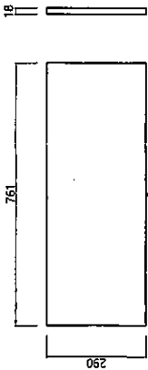
이동선반 가공도
