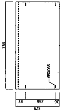
천판 가공도
