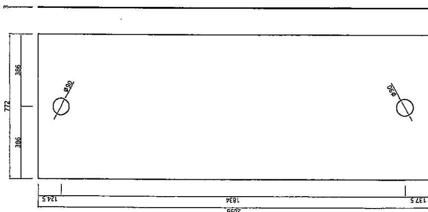
뒷판 가공도
