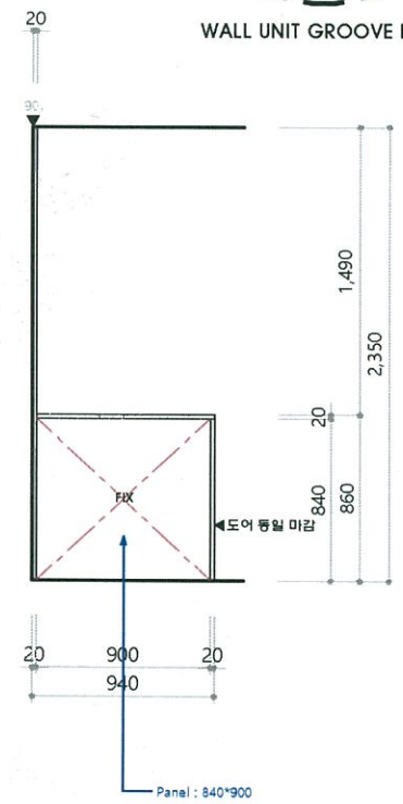
ELEVATION - C''
